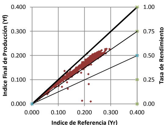
Indice Final de Producción Vs Indice de Referencia Monocristalino 2 - NOVIEMBRE
