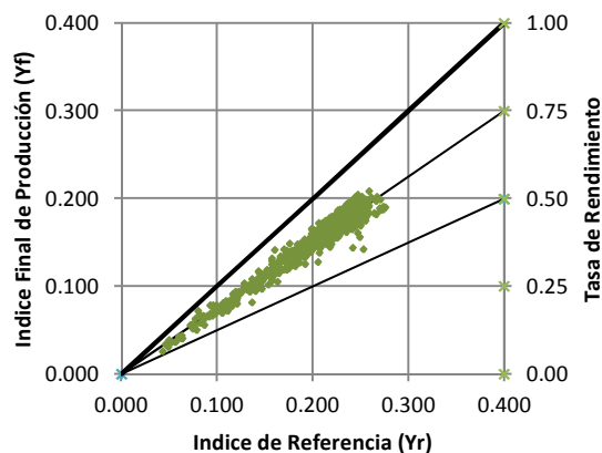
Indice Final de Producción Vs Indice de Referencia Amorfo 1 - ENERO
