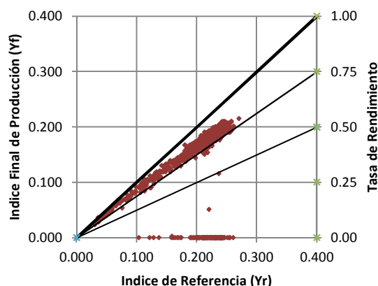
Indice Final de Producción Vs Indice de Referencia Monocristalino 2 - DICIEMBRE
