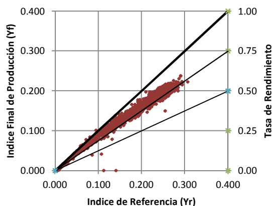
Indice Final de Producción Vs Indice de Referencia Monocristalino 2 - OCTUBRE
