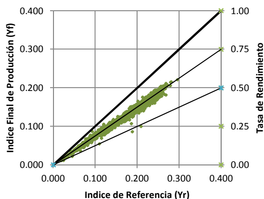
Indice Final de Producción Vs Indice de Referencia Amorfo 1 - ABRIL
