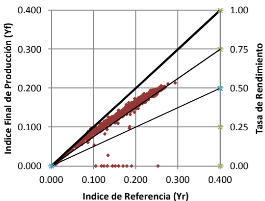
Indice Final de Producción Vs Indice de Referencia Monocristalino 2 - JULIO
