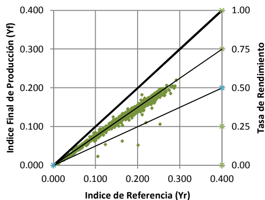
Indice Final de Producción Vs Indice de Referencia Amorfo 1 - JUNIO
