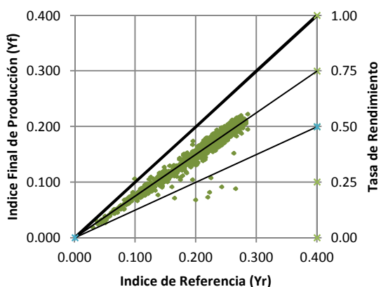
Indice Final de Producción Vs Indice de Referencia Amorfo 1 - MARZO
