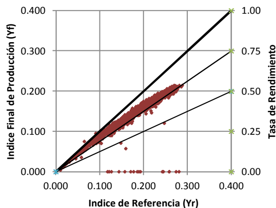
Indice Final de Producción Vs Indice de Referencia Monocristalino 2 - AGOSTO
