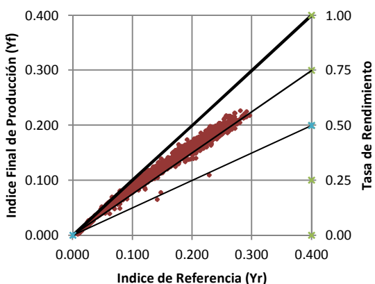
Indice Final de Producción Vs Indice de Referencia Monocristalino 2 - SEPTIEMBRE
