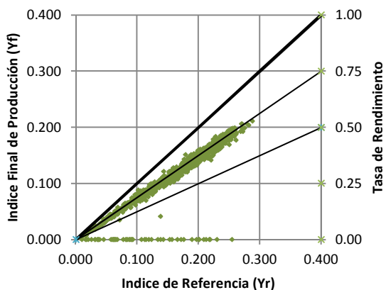
Indice Final de Producción Vs Indice de Referencia Amorfo 1 - MAYO
