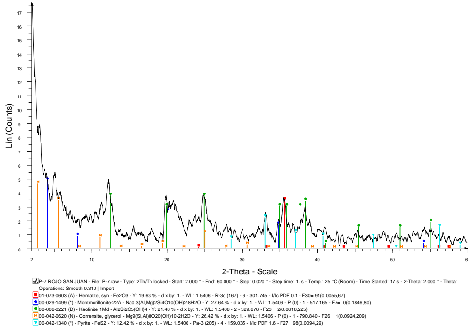
Figura N. 39: DIFRACTOGRAMA muestra color rojo San Juan
