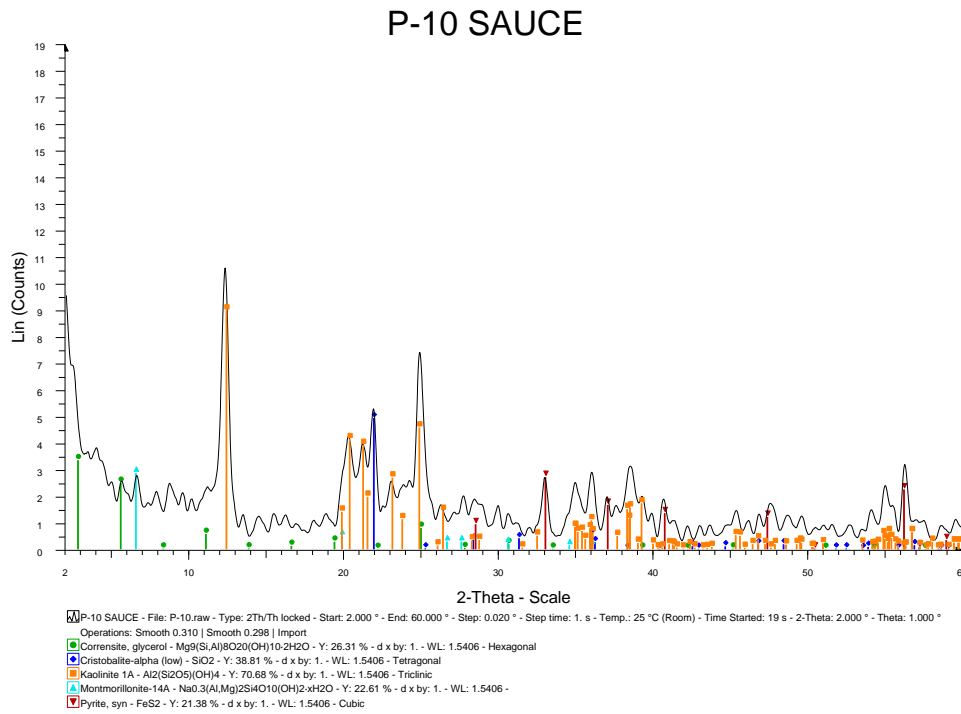
Figura N. 41: DIFRACTOGRAMA muestra color Café El Sauce
