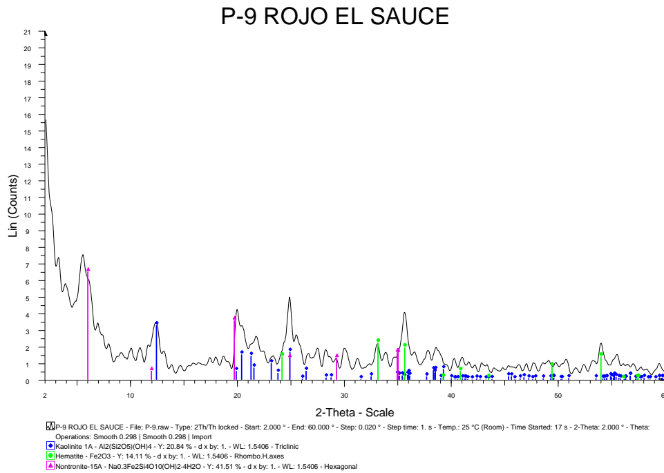
Figura N. 40: DIFRACTOGRAMA muestra color rojo El Sauce
