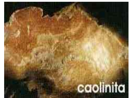
Figura No 30 Caolinita
