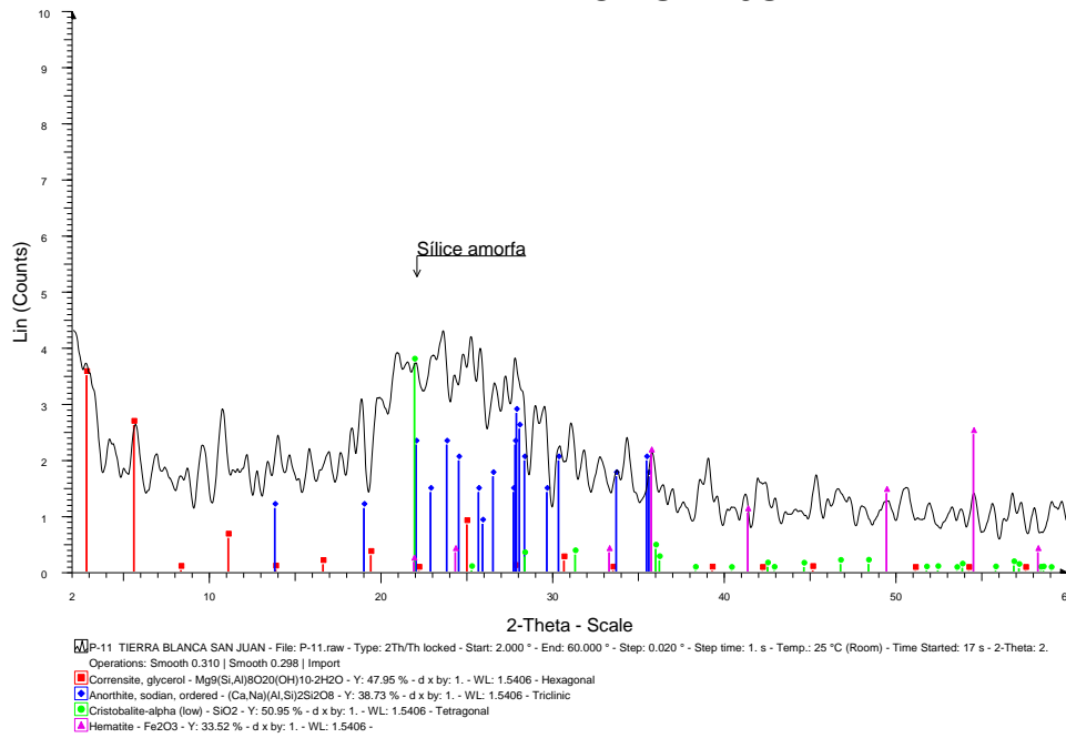
Figura N. 42: DIFRACTOGRAMA muestra tierra blanca San Juan
