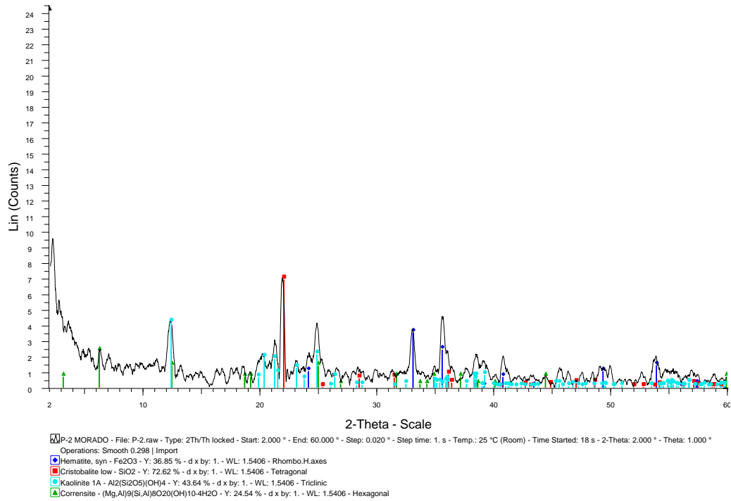
Figura N. 38: DIFRACTOGRAMA muestra color morado
