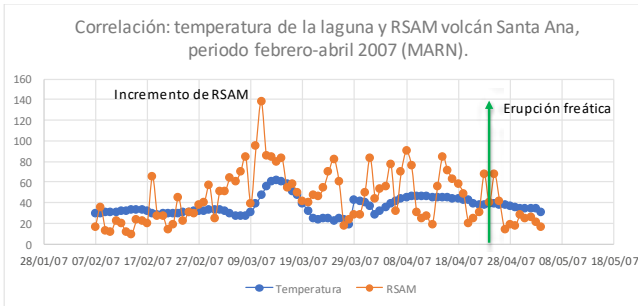
Figura 4. Comportamiento de RSAM y temperatura de la laguna del volcán Santa Ana, febrero-abril 2007 (MARN, 2007).
