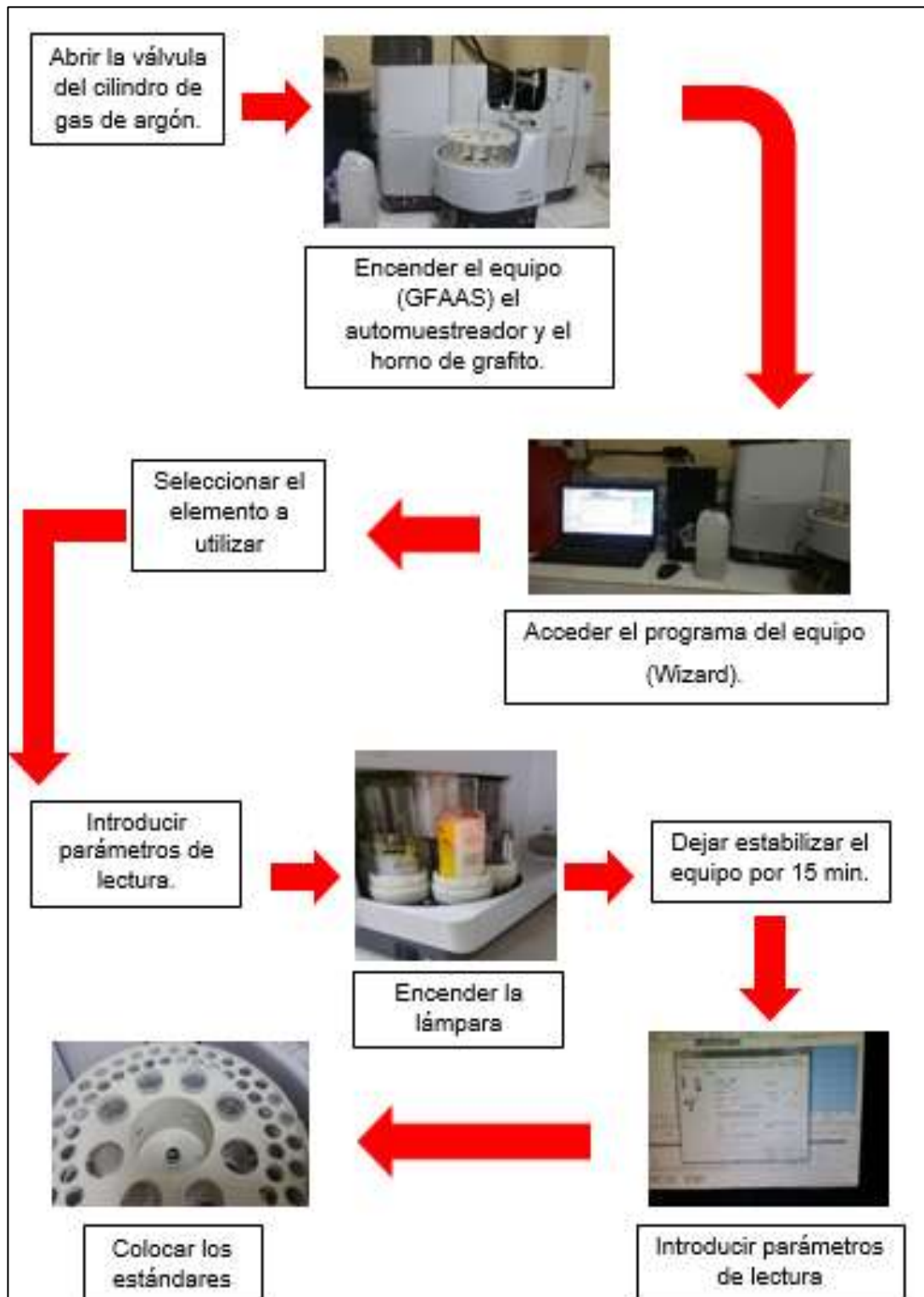
Figura N°17: Procedimiento para la cuantificación de Plomo
