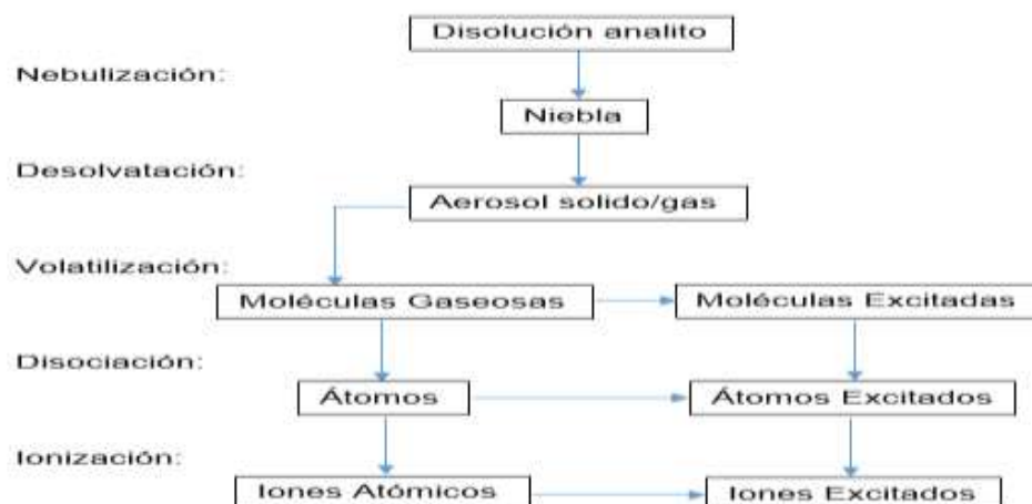
Figura N°3: Espectroscopia de absorción atómica. Procesos durante la Atomización. (17)
