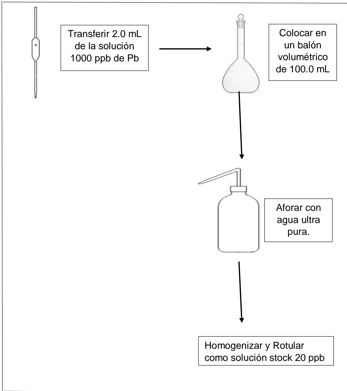
Figura N°18: Esquema de dilución de la solución stock.
