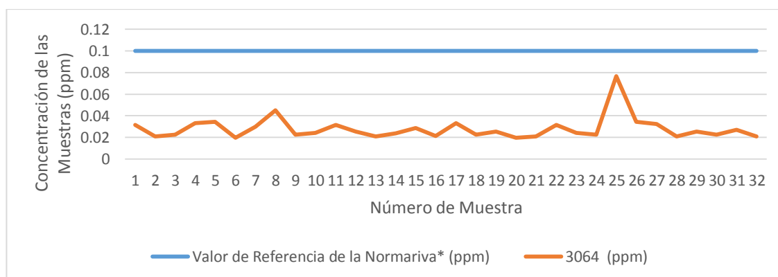
Figura N°6: Gráfica de las concentraciones de Plomo (ppm) en 32 muestras de Lycopersicon esculentum (Tomate) de la variedad o zona de cultivo (3064) por el método de espectroscopia de Absorción Atómica con
