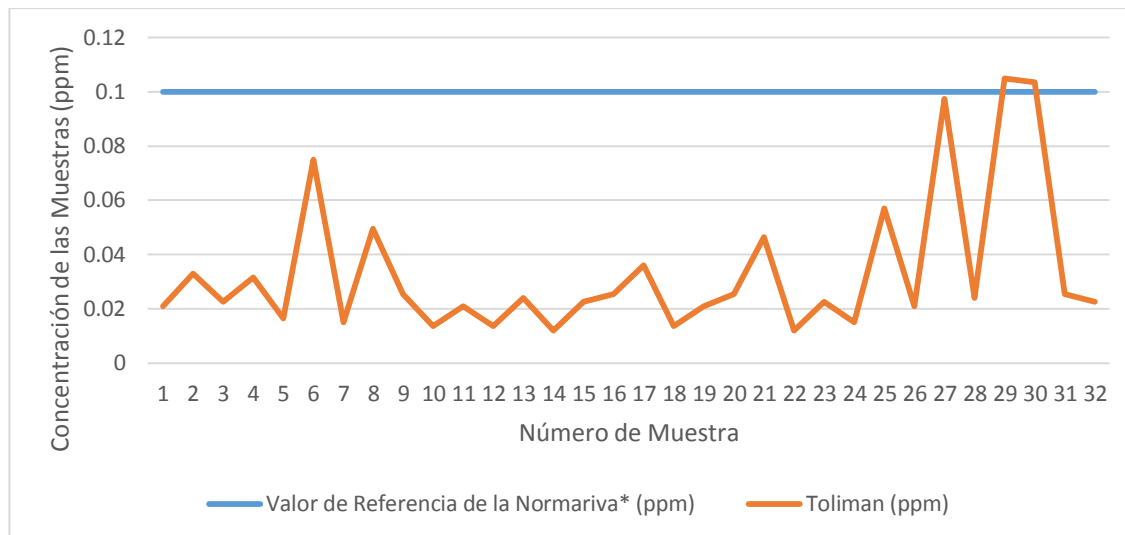
Figura N°7: Gráfica de las concentraciones de Plomo (ppm) en 32 muestras de Lycopersicon esculentum (Tomate) de la variedad o zona de cultivo (Toliman) por el método de espectroscopia de Absorción Atómica con
