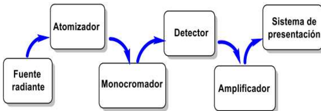
Figura N° 4: Los principales componentes de un Espectrofotómetro de Absorción Atómica.
