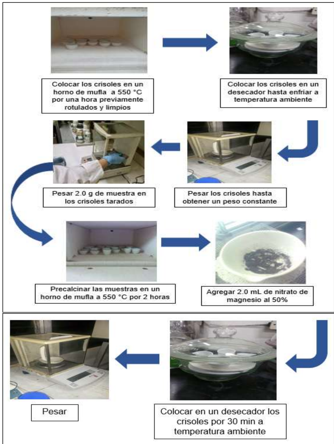
Figura N° 15: Incineración por secado.
