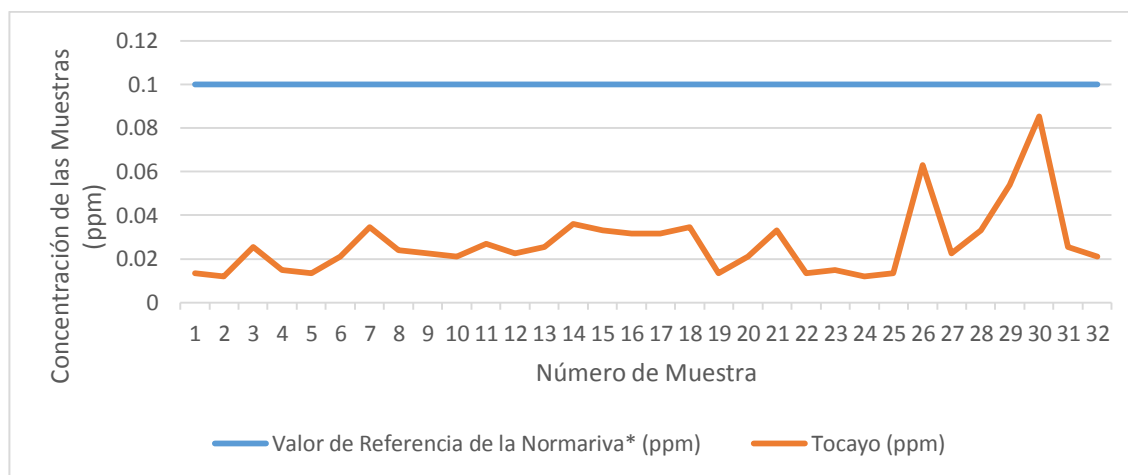
Figura N°8: Gráfica de las concentraciones de Plomo (ppm) en 32 muestras de Lycopersicon esculentum (Tomate) de la variedad o zona de cultivo (Tocayo) por el método de espectroscopia de Absorción Atómica con Horno de Grafito.
