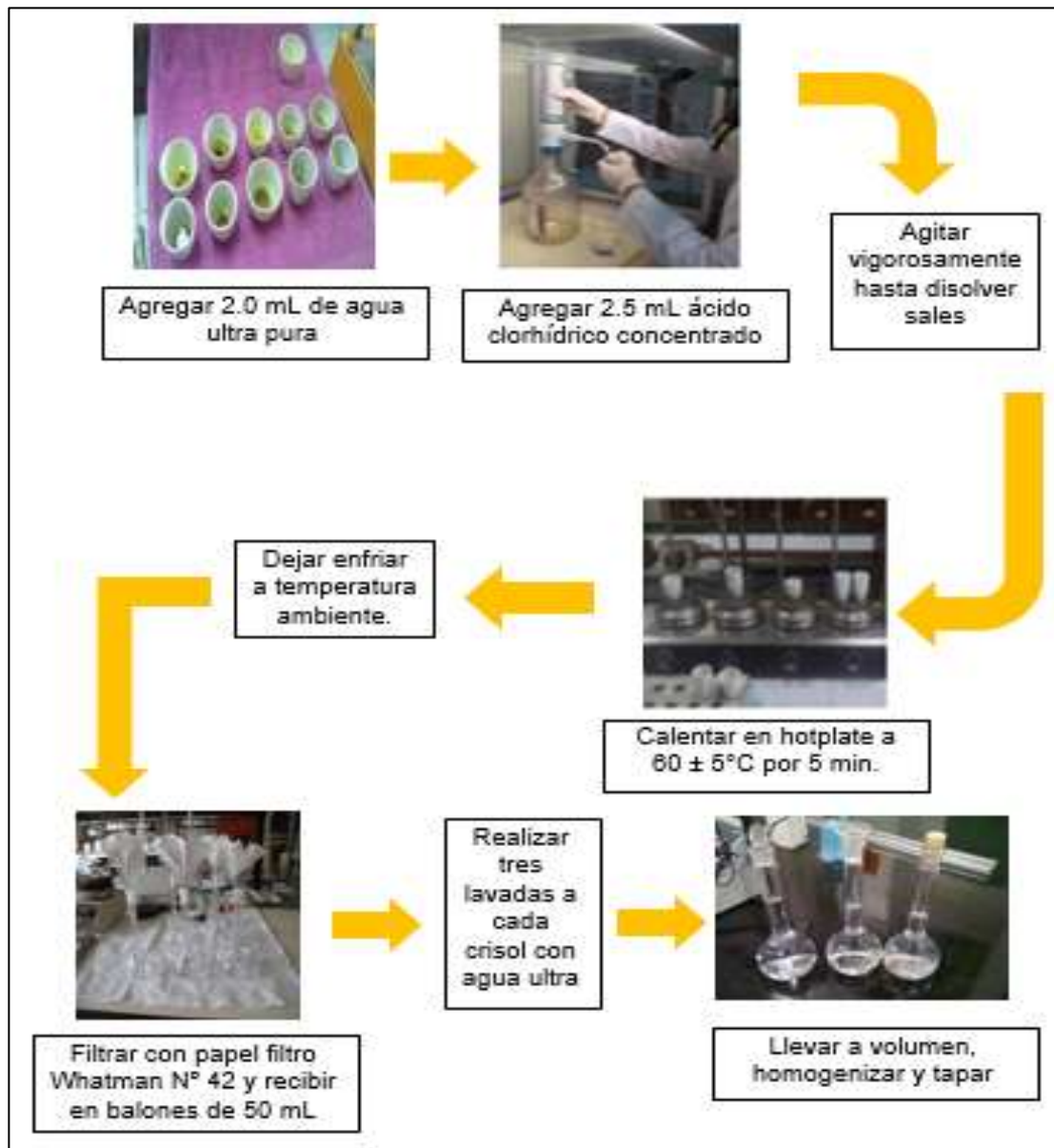
Figura N° 16: Preparacion de soluciones madre.
