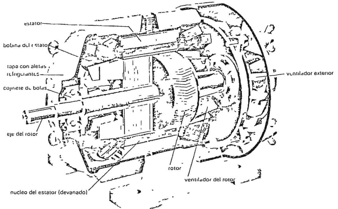
Motor trifasico
