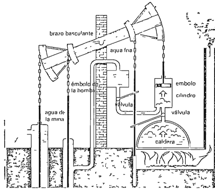
Maquina de vapor de Newcomen
