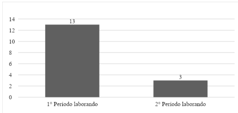
Figura 3: Resultados pregunta 1
