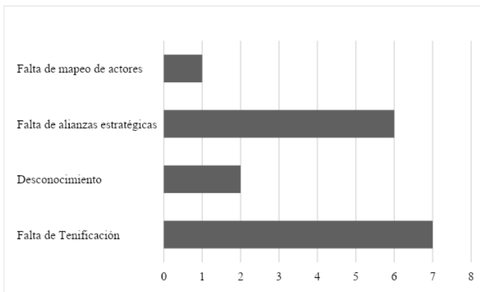
Figura 9: Resultados pregunta 7
