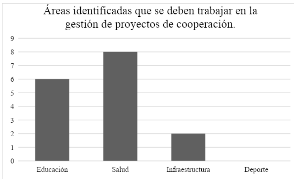
Figura 10: Resultados pregunta 8
