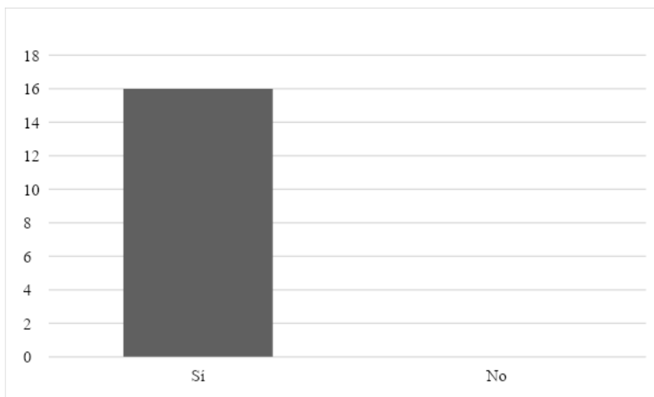
Figura 8: Resultados pregunta 6
