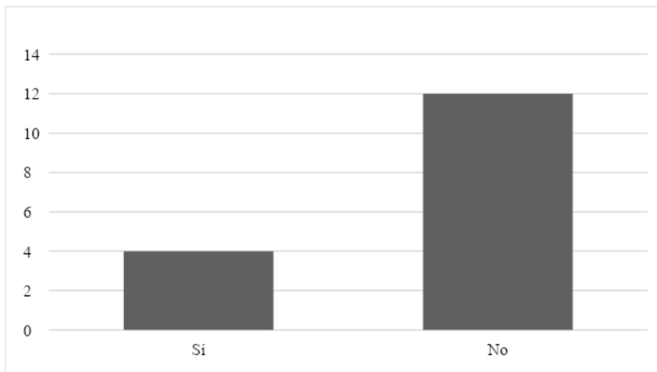
Figura 5: Resultados pregunta 3
