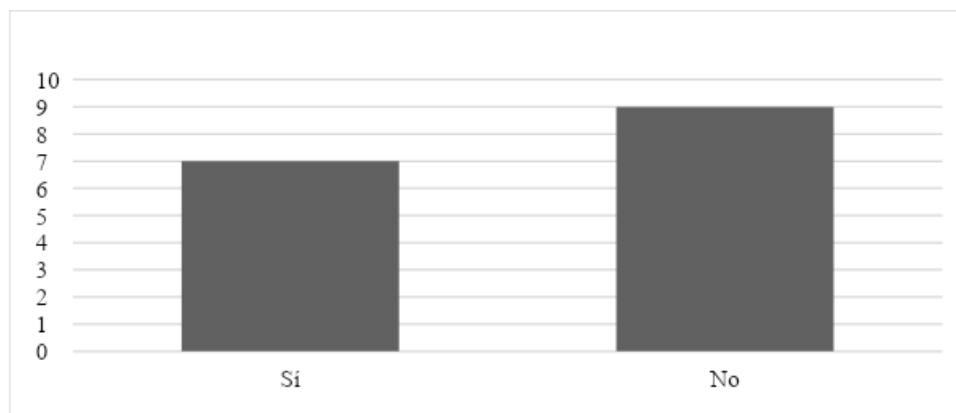
Figura 4: Resultados pregunta 2
