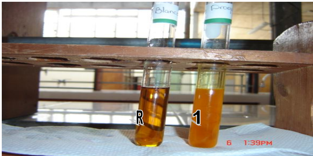
FIG N° 23: Prueba para alcaloides Referencia (R) y Dragendorff (1)
