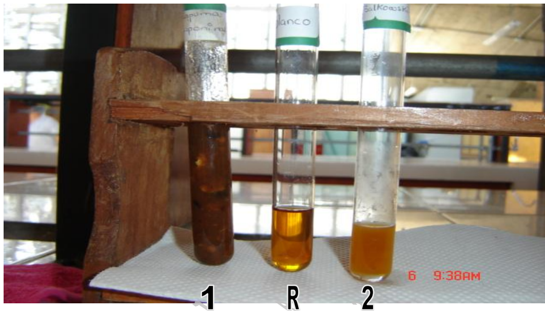
FIG N°19: Resultados de pruebas cualitativas para saponinas: prueba de la espuma (1), Referencia (R) y Salkowski (2)
