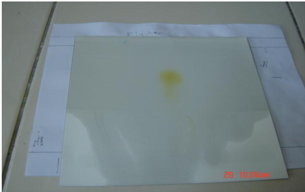
FIG N°28: Localizacion de flavonoides en la placa cromatográfica.
