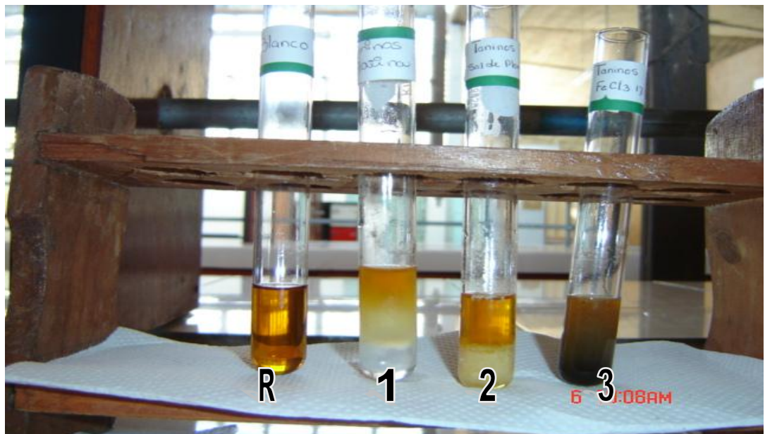
FIG Nº 21: Resultados de pruebas de identificación de taninos Referencia (R), Gelatina (1), Acetato de plomo (2) tricloruro de hierro (3)
