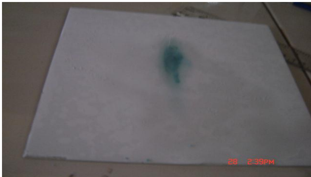
FIG N°27: Localización de Saponinas en la placa cromatográficas
