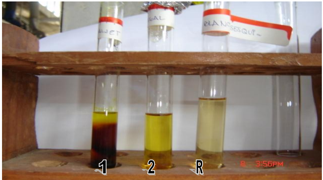
FIG N° 22: Resultados de pruebas de identificación de sesquiterpenolactonas: Baljet (1), Legal (2) y Referencia (R)
