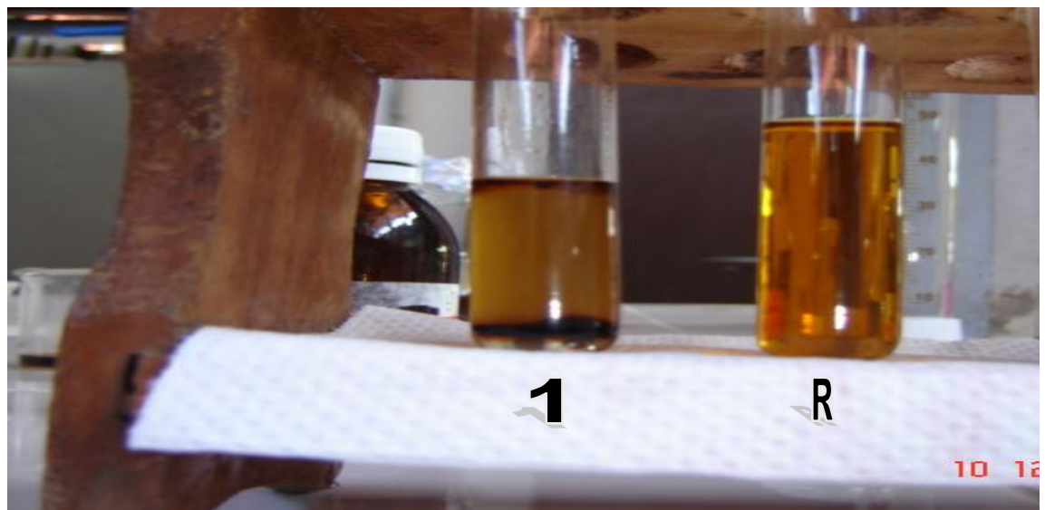
FIG N° 25 : Resultados de la prueba de Liebermann Buchard (1) y Referencia (R)
