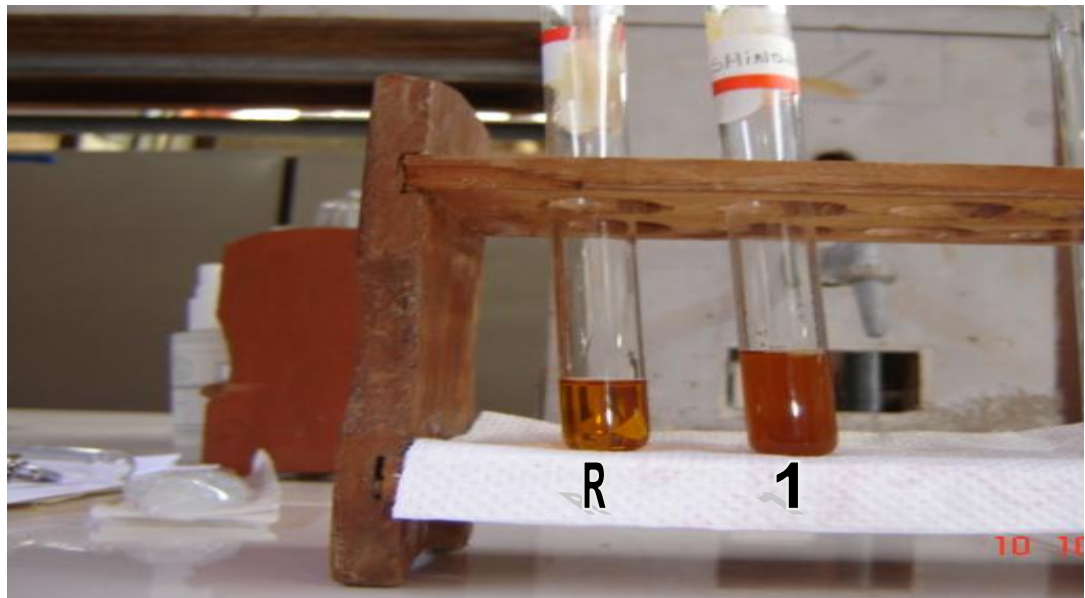
FIG Nº20 : Resultados de la prueba de Shinoda para flavonoides (1) y Referencia (R)
