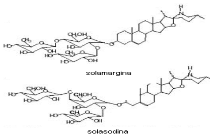
FIG N° 3: Estructuras de alcaloides esteroidales
