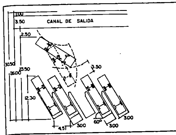
PLATAFORMA DE ASCENSO ALTERNATIVA A 60°
