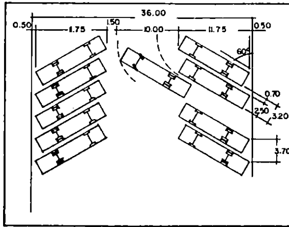
ESTACIONAMIENTO DOBLE ALTERNATIVA A 60°.
