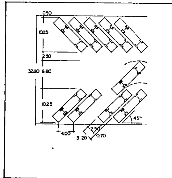
ESTACIONAMIENTO DOBLE ALTERNATIVA A 45°
