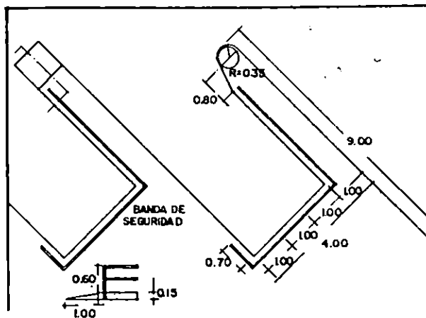
DETALLE DE UNA PLATAFORMA DENTADA A 45°
