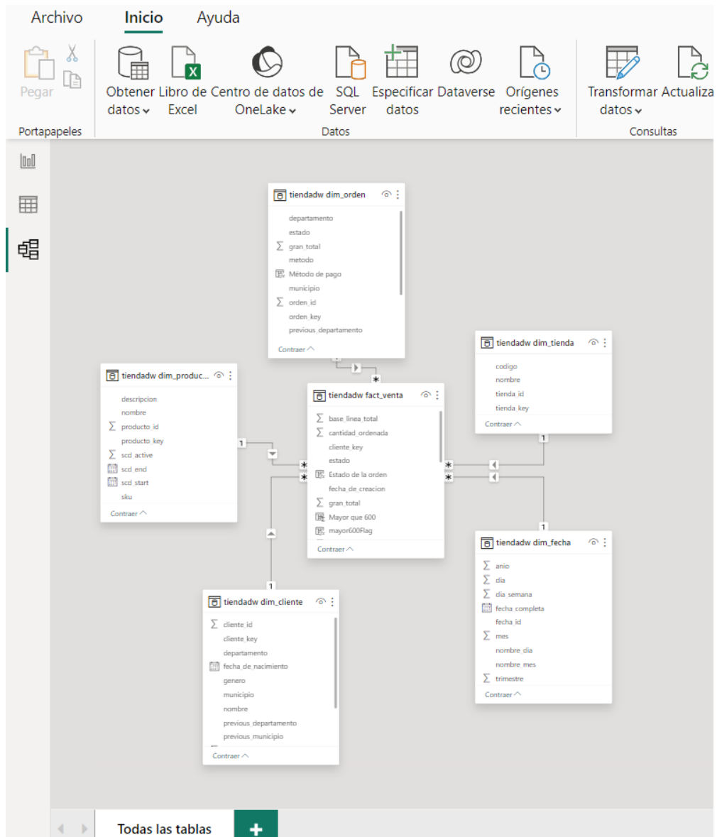
Ilustración 23. Modelo de estrella cargado en PowerBI
