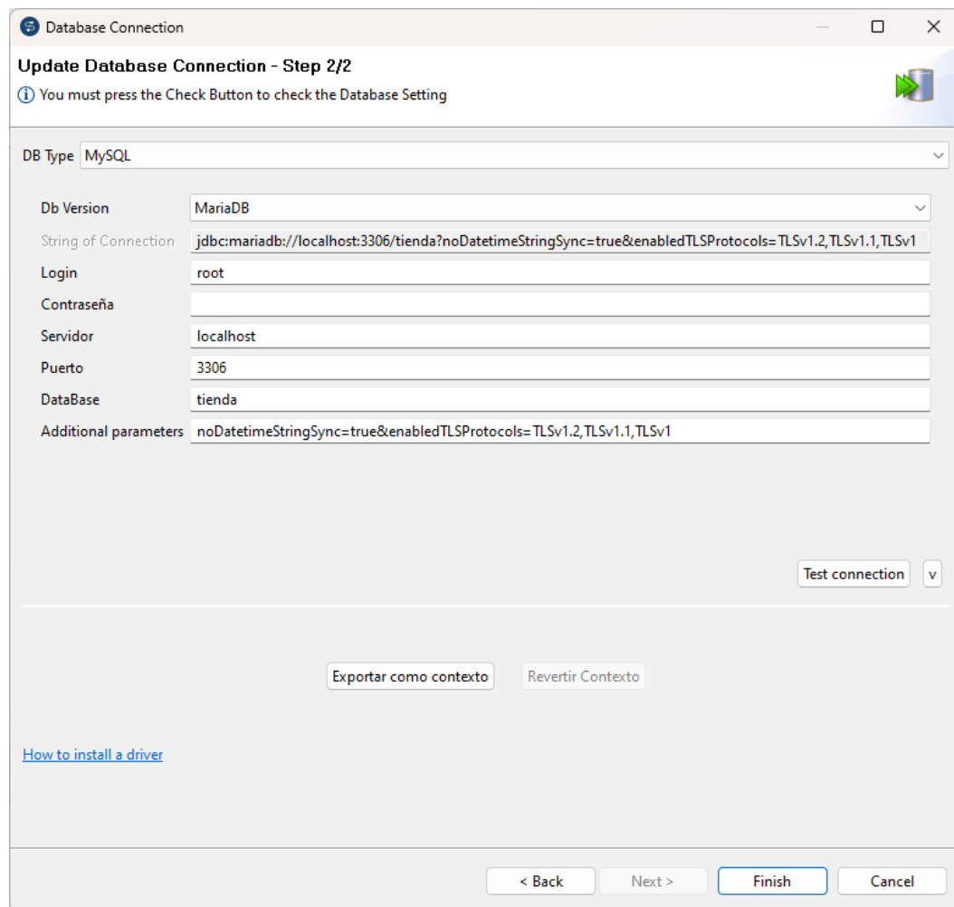
Ilustración 11. Configurar credenciales de acceso
