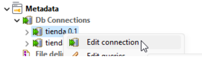
Ilustración 10. Editar conexión
