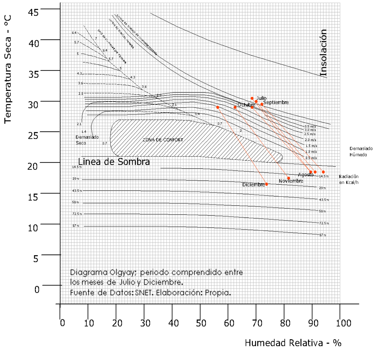
Imagen No. 32 Diagrama de Olgyay. Julio - Diciembre
