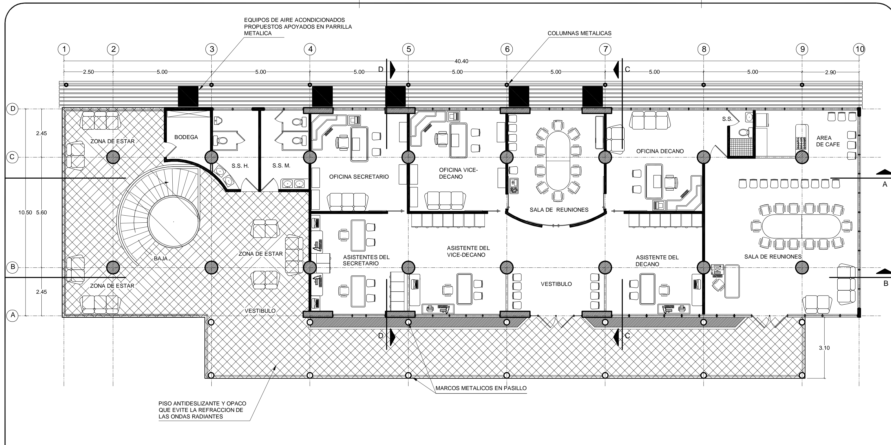
PLANTA ARQUITECTONICA PROPUESTA - NIVEL 3 ESC. 1:100
