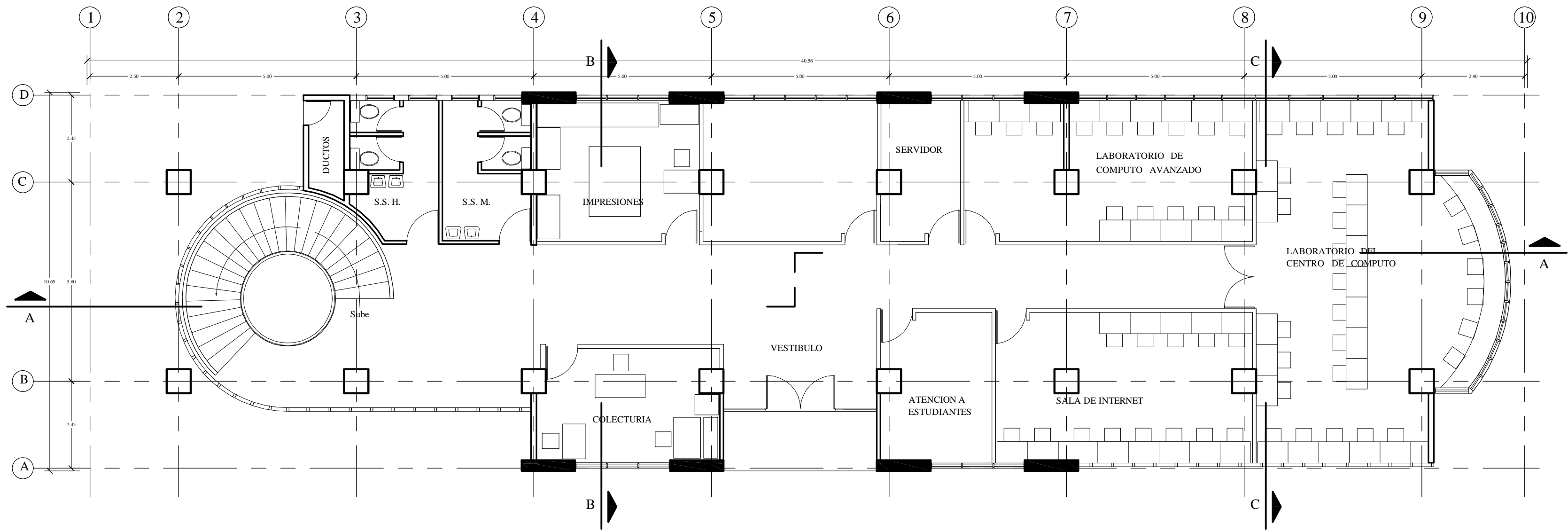
PLANTA ARQUITECTONICA EXISTENTE - NIVEL 1 NPT = 0 +0.00 ESC. 1:100
