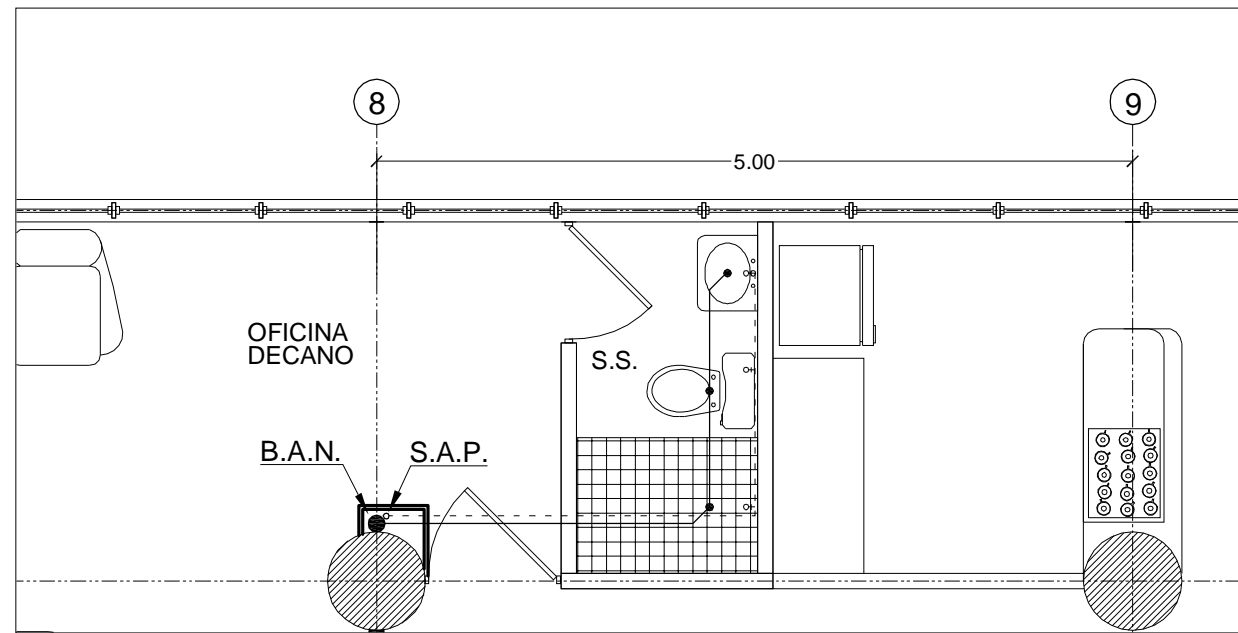
RED HIDRAULICA EN SANITARIO PROPUESTO DECANATO - NIVEL 3 ESC. 1:50
