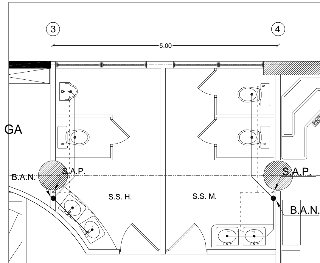
RED HIDRAULICA SANITARIOS EN LOS 3 NIVELES ESC. 1:50
