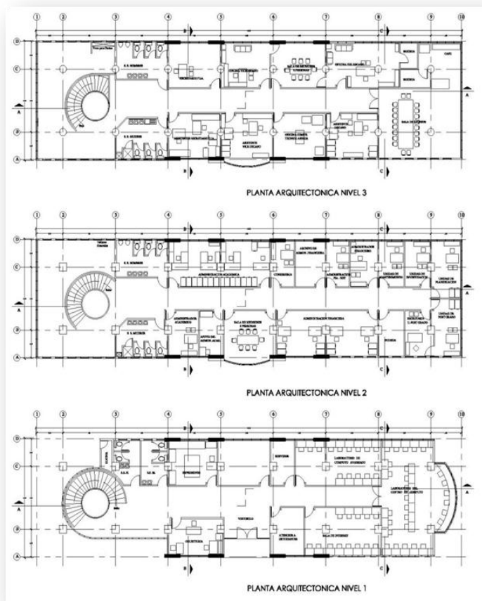
Imagen No. 30 Distribución Arquitectónica Actual. Fuente: Unidad de Desarrollo Físico.
