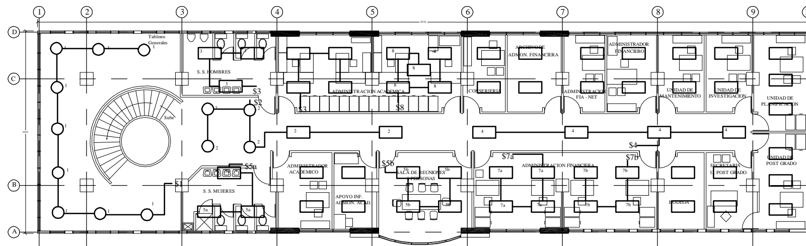
PLANTA DE LUMINARIAS NIVEL 2 NPT = 0 +4.30 SIN ESCALA
