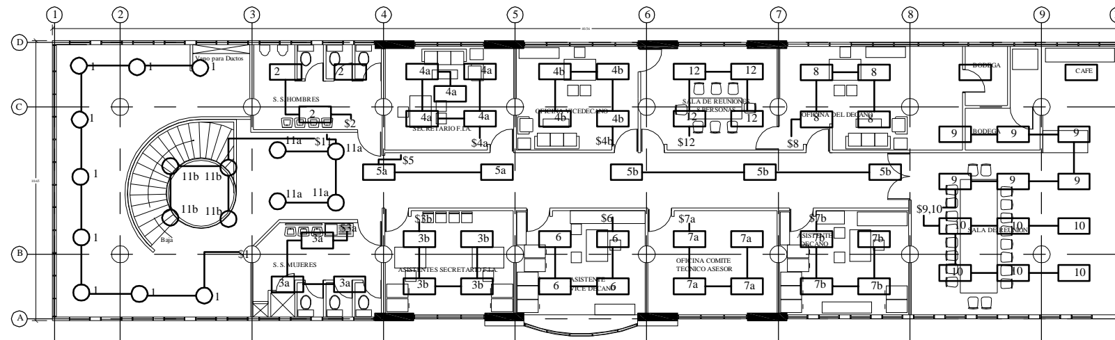
PLANTA DE LUMINARIAS NIVEL 3 NPT = 0 +7.80 SIN ESCALA
