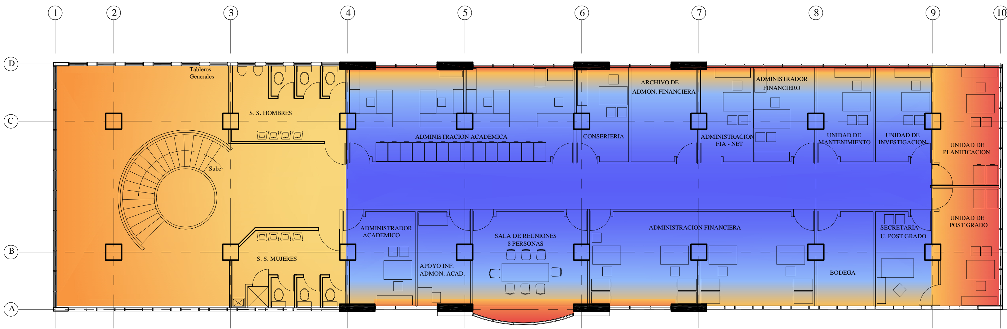
AMBIENTE TERMICO EXISTENTE - NIVEL 2 NPT = 0 +4.30 ESC. 1:100
