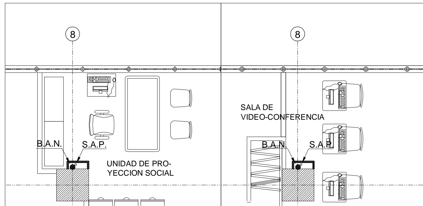
SUBIDA DE AGUA POTABLE Y BAJADA DE AGUAS NEGRAS NIVELES 1 Y 2 ESC. 1:50
