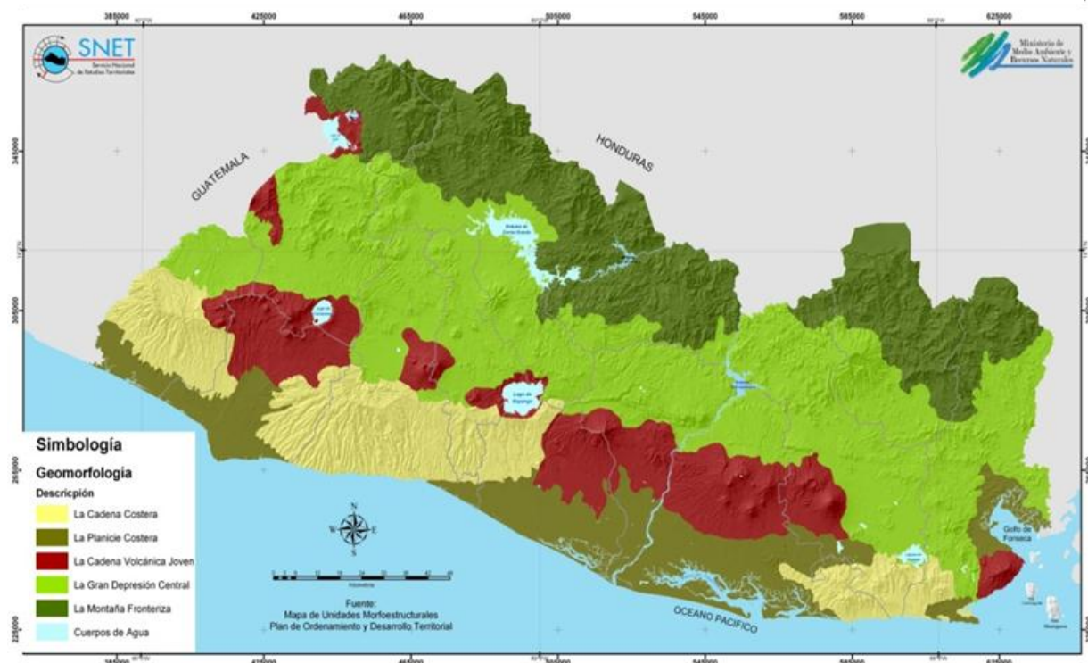
Imagen No. 6 Mapa Geomorfológico de El Salvador
