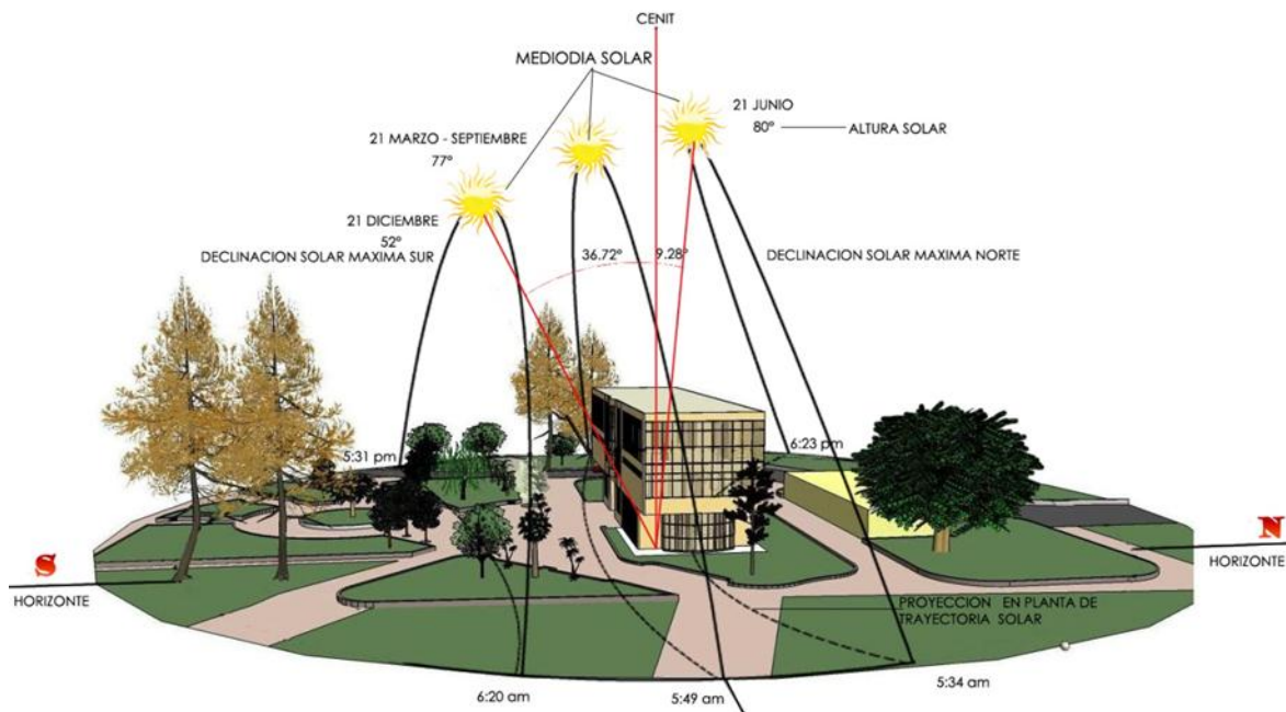
Imagen No. 34 Trayectoria Solar
