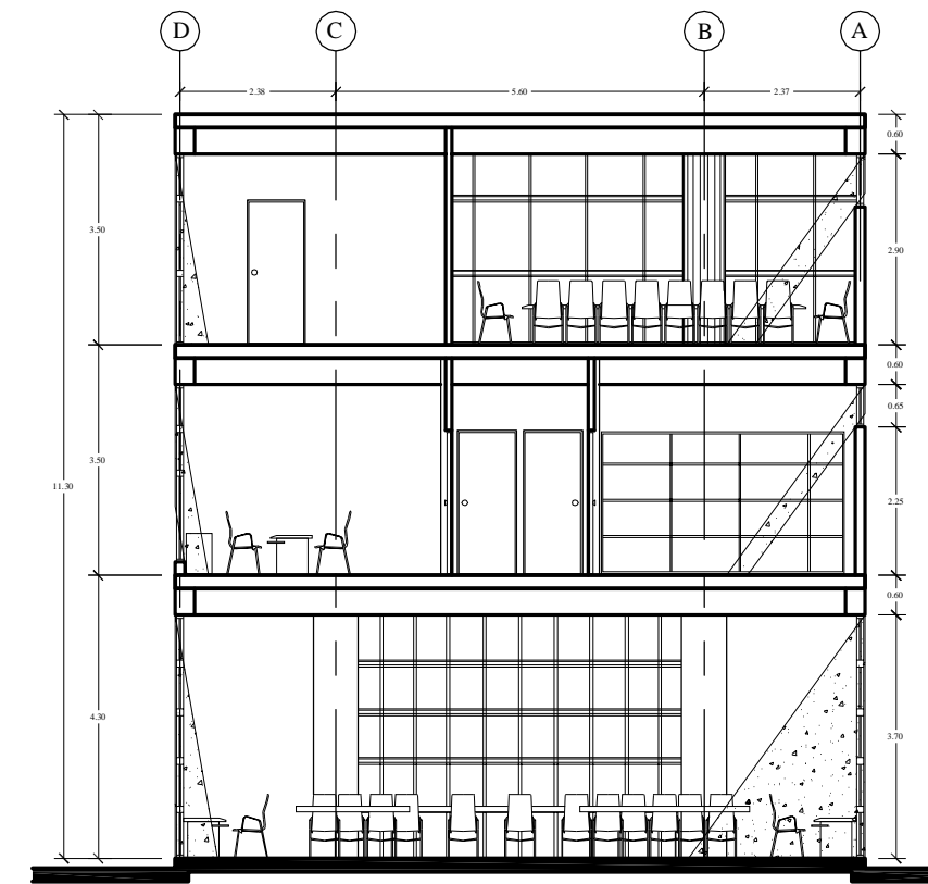
SECCION C-C ESC. 1:125
