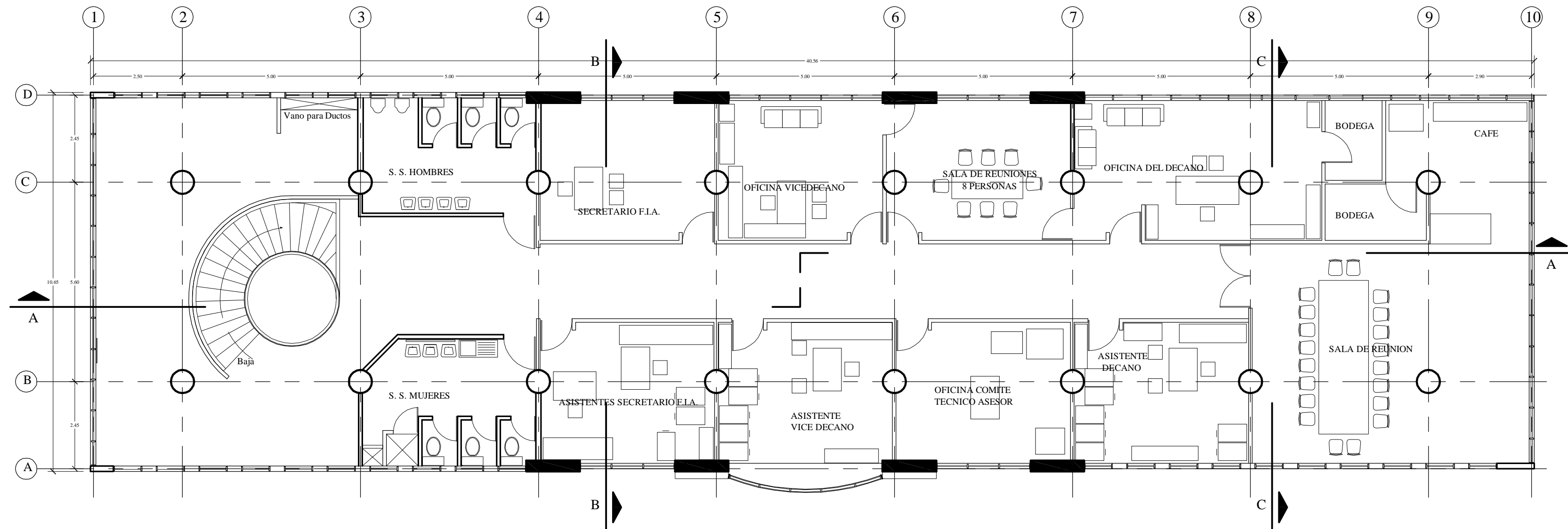
PLANTA ARQUITECTONICA EXISTENTE - NIVEL 3 NPT = 0 +7.80 ESC. 1:100
