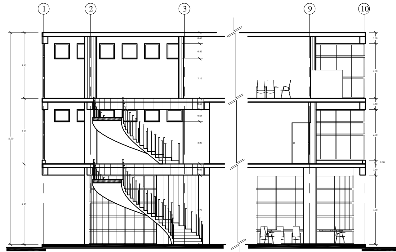
SECCION A-A ESC. 1:125
