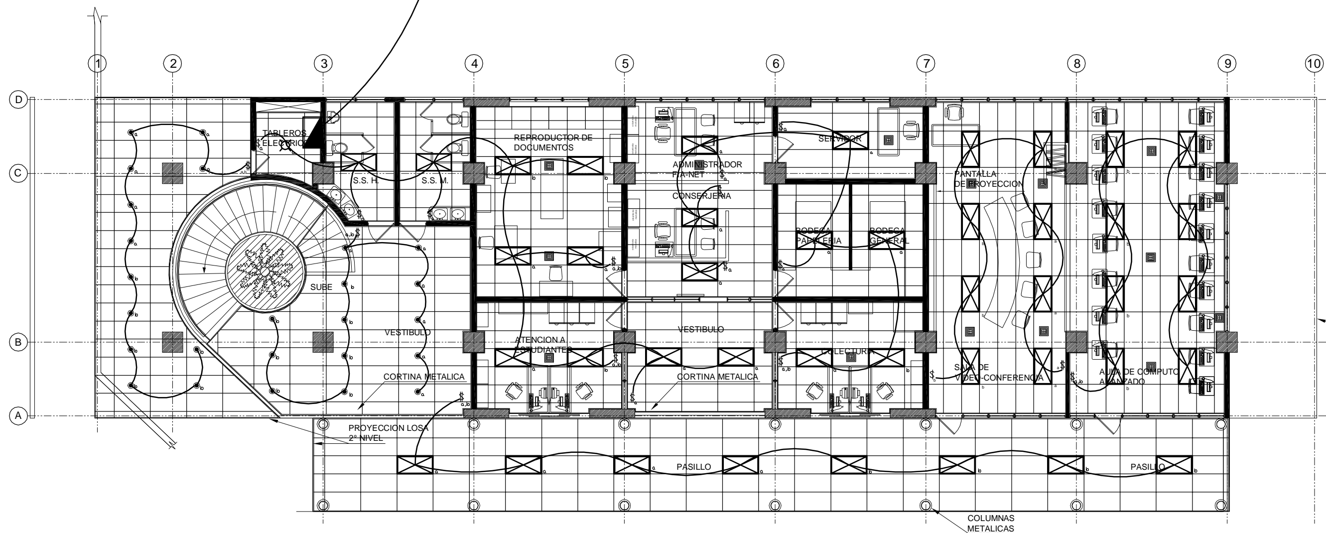
PLANTA DE CIELO REFLEJADO Y LUMINARIAS NIVEL 1 ESC. 1:125
