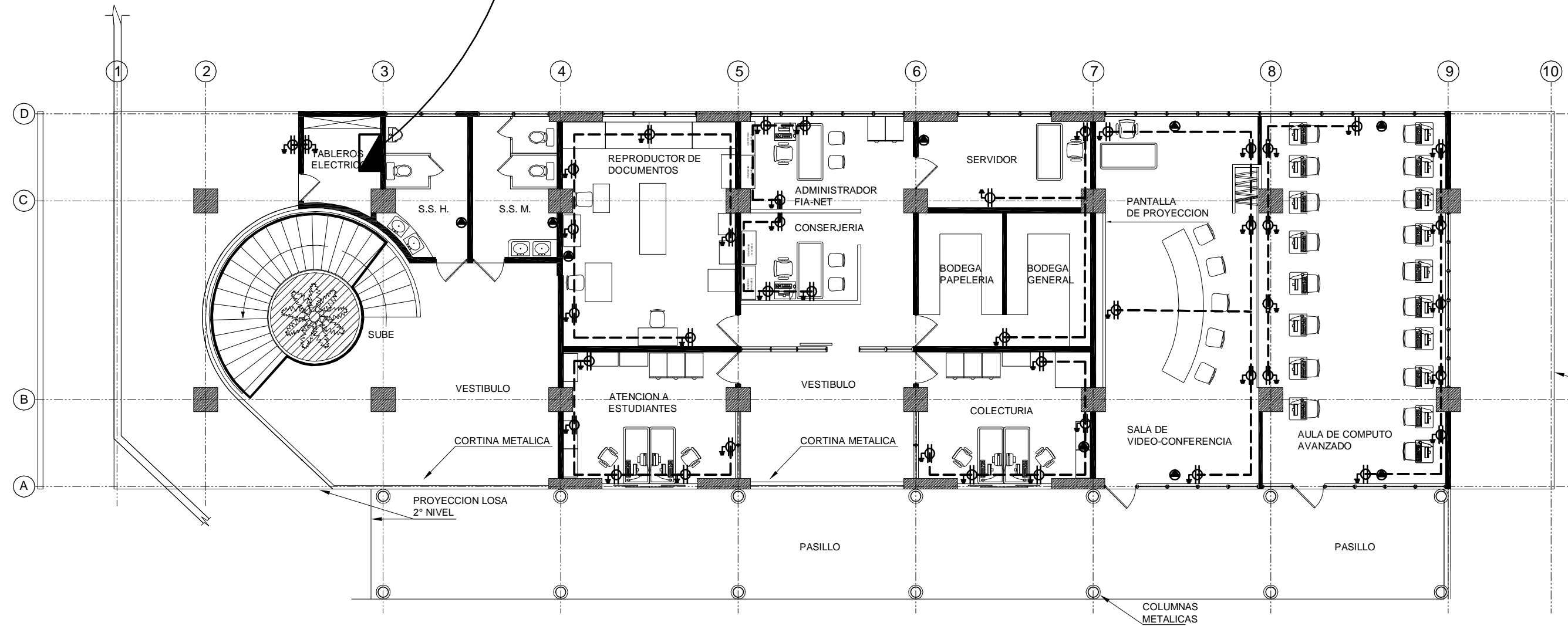
PLANTA DE TOMACORRIENTES NIVEL 1 ESC. 1:125
