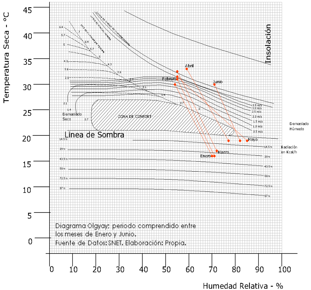
Imagen No. 31 Diagrama de Olgay. Enero - Junio
