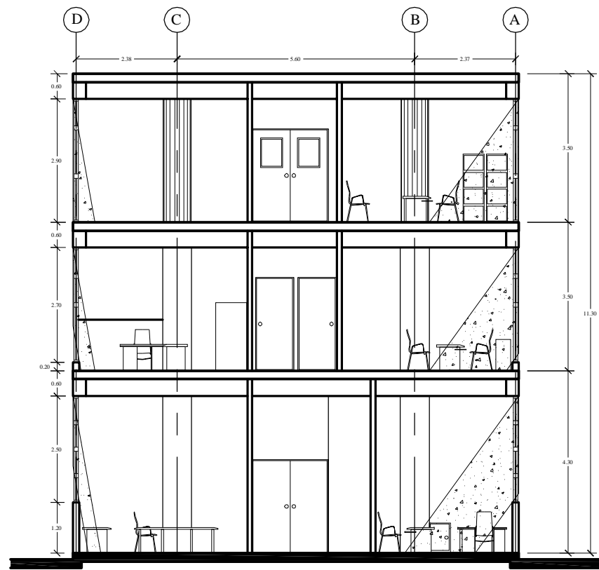
SECCION B-B ESC. 1:125
