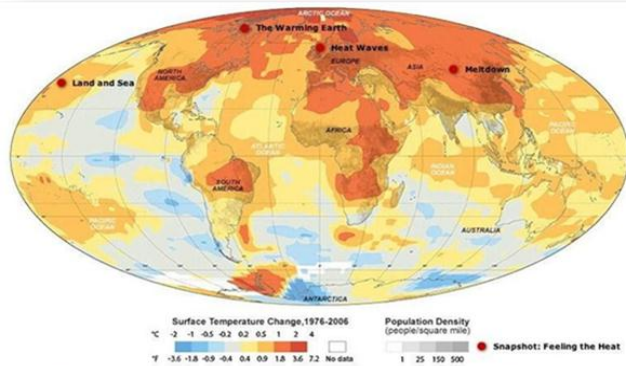
Imagen No. 9 Variación de la Temperatura Global: 1976 - 2006
