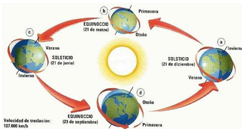
Imagen No. 12 Rotación y Traslación de la Tierra alrededor del Sol.
