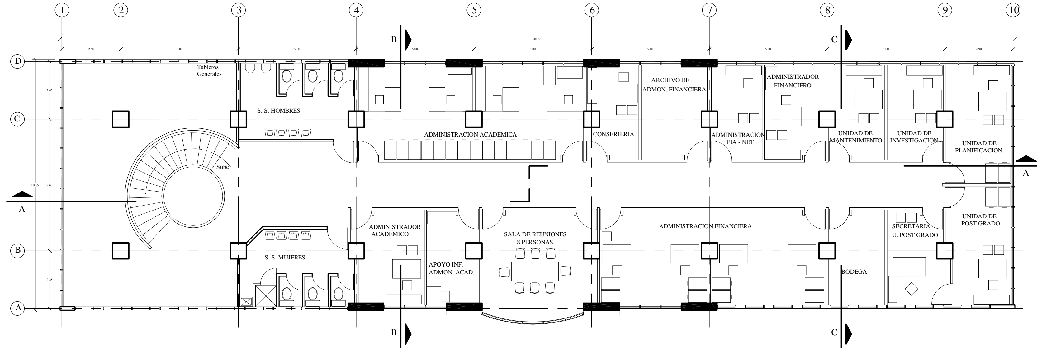
PLANTA ARQUITECTONICA EXISTENTE - NIVEL 2 NPT = 0 +4.30 ESC. 1:100
