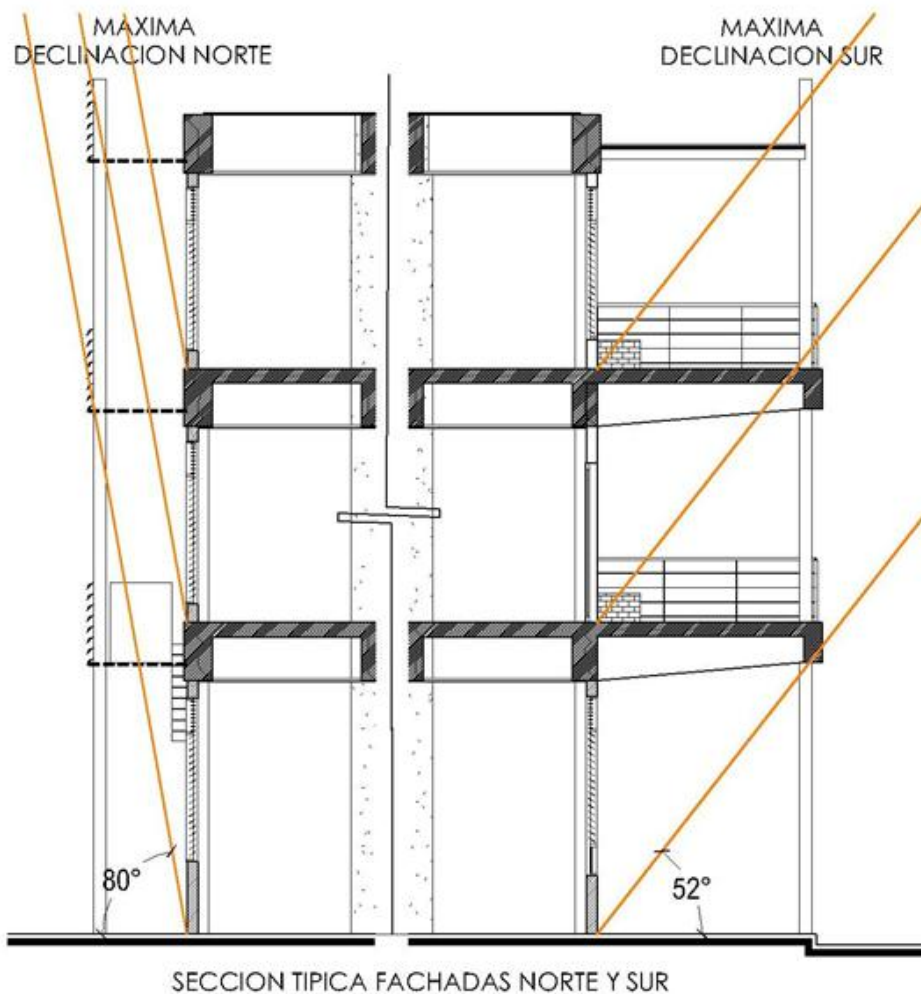
Imagen No. 35 Incidencia Solar sobre fachadas Norte y Sur
