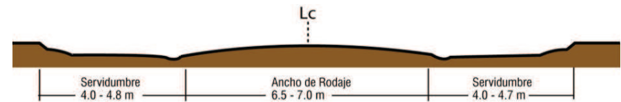
Sección de Carretera a Quezaltepeque
