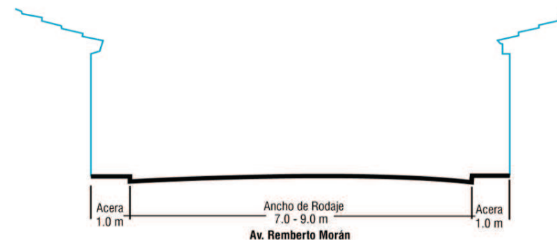
Sección de Vía Primaria
