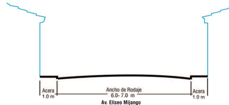
Sección de Vía Secundaria
