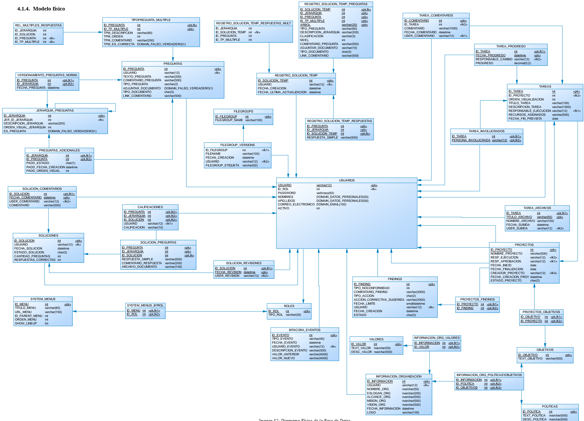
Imagen 32: Diagrama Físico de la Base de Datos
