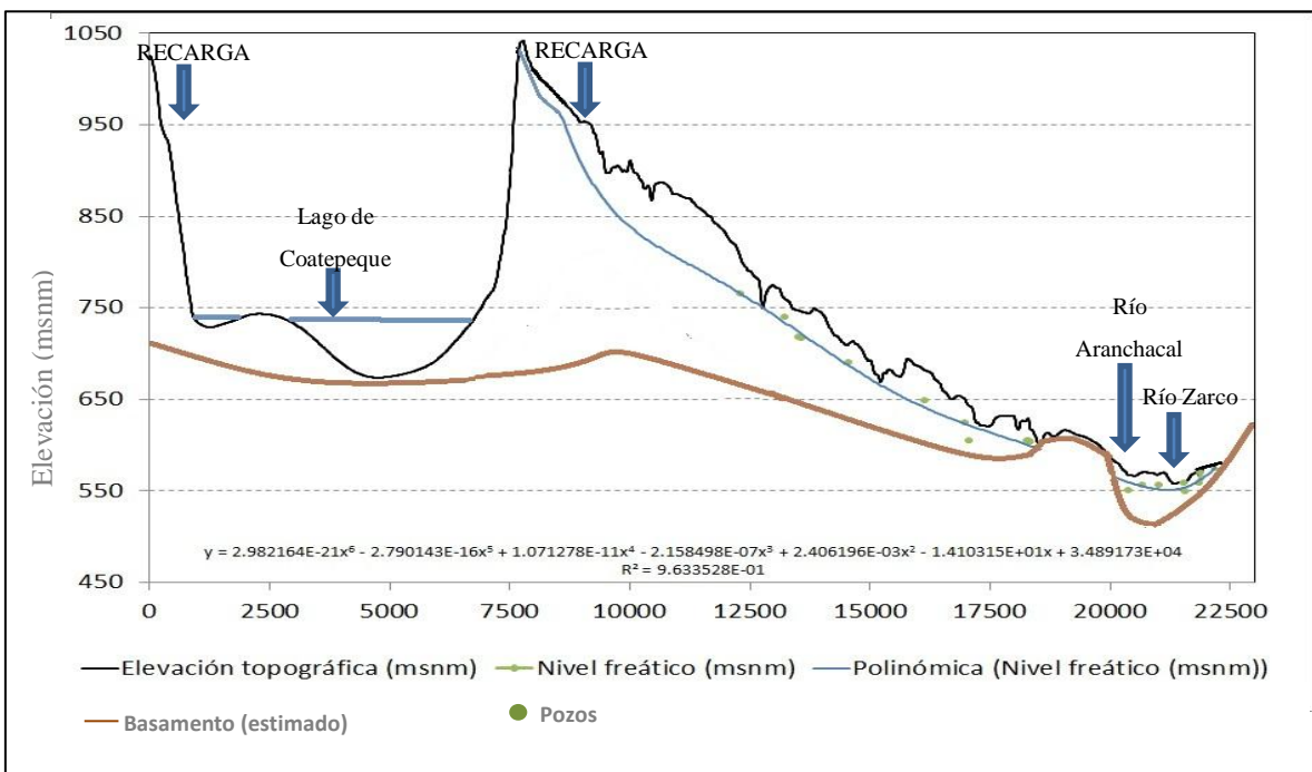
Figura 153 Corte de perfil CD Fuente: Elaboración propia.
