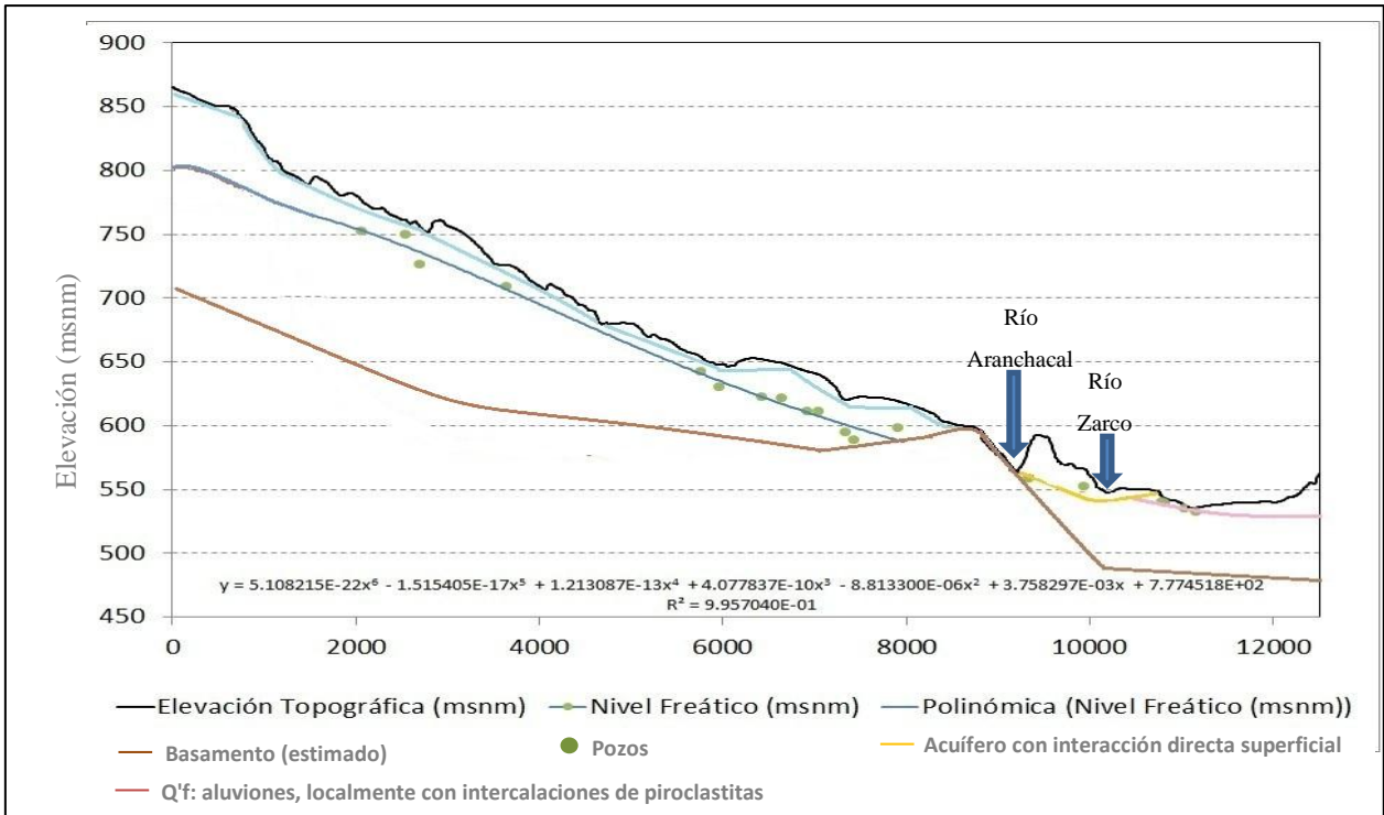
Figura 152 Corte de Perfil AB Fuente: Elaboración propia.
