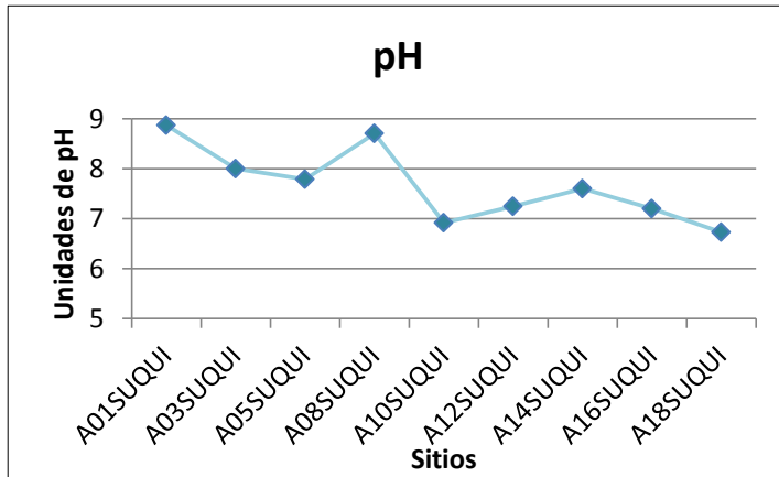
Figura 45 Gráfica de pH medido a lo largo del río Suquia
