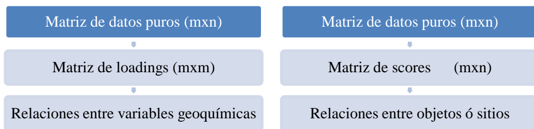
Figura 11 Esquema de cálculo de componentes principales.
