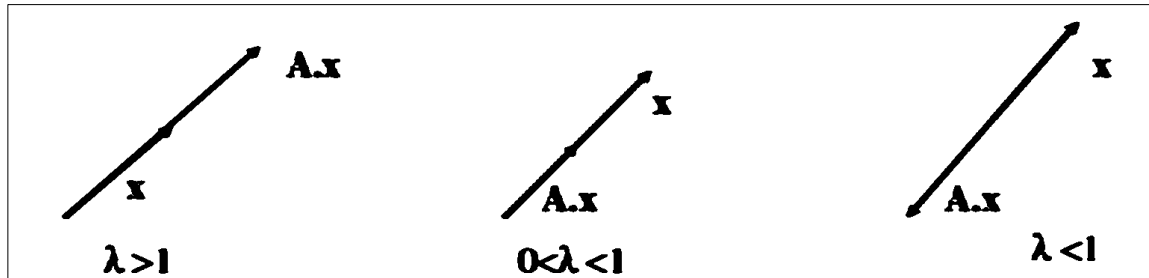
Figura 13 Esquema de eigenvalues en el espacio
