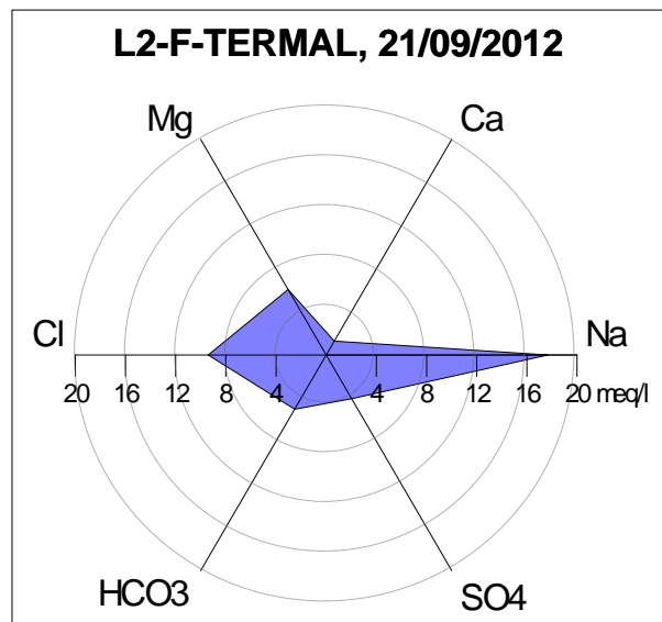
Figura 65 Ejemplo de gráfico radial de composición de especies mayoritarias del sitio: Fuente termal del Lago de Coatepeque
