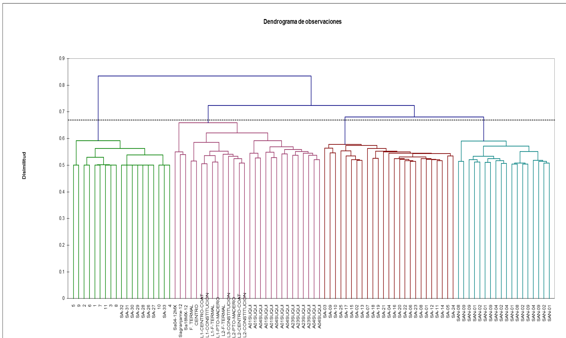
Figura 129 Dendrogramas de sitios de muestreo de la base de datos geoquímica del área geográfica de interés
