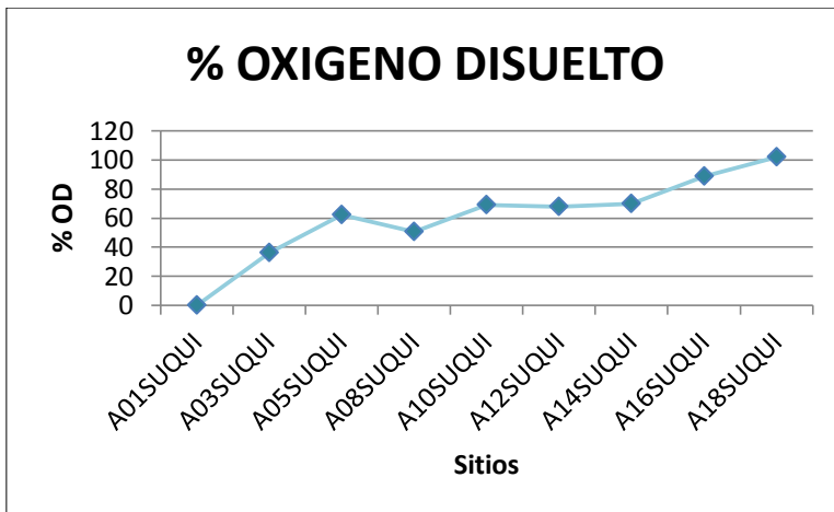
Figura 46 Valores de porcentaje de Oxígeno Disuelto a lo largo del río Suquia
