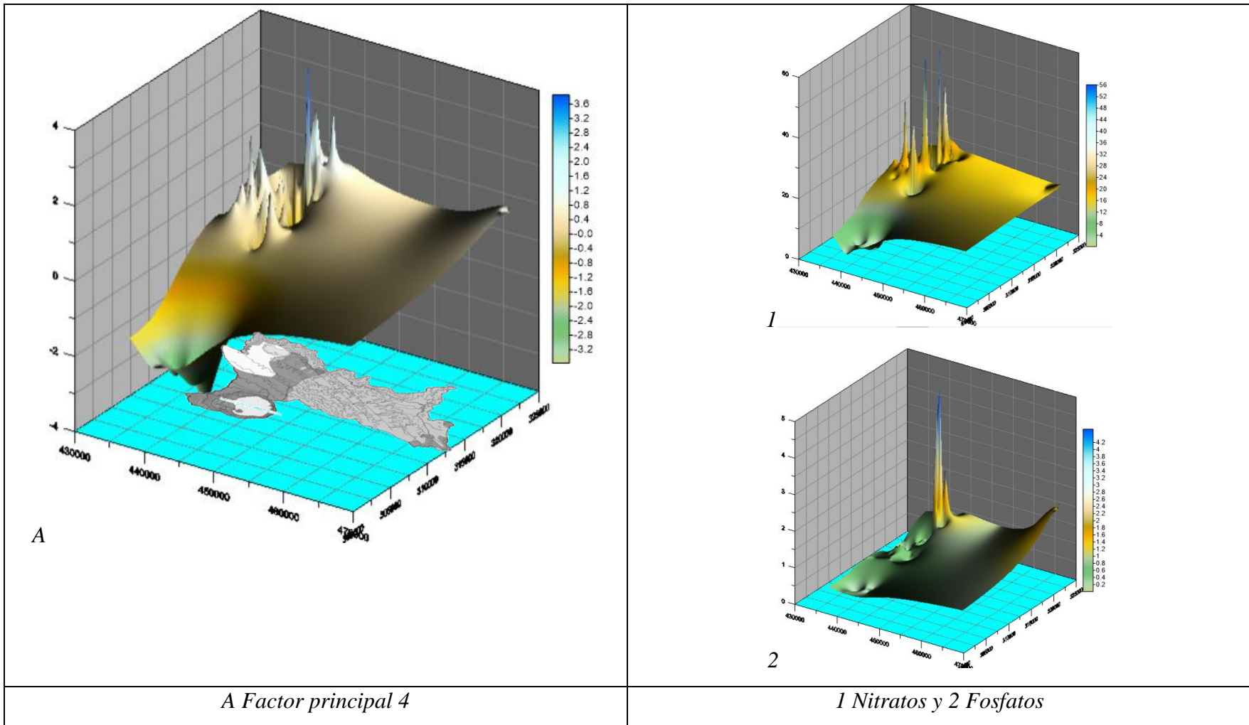
Figura 113 Comparación gráfica entre las superficies paramétricas del componente principal 4 y algunas especies químicas Fuente: Elaboración propia.
